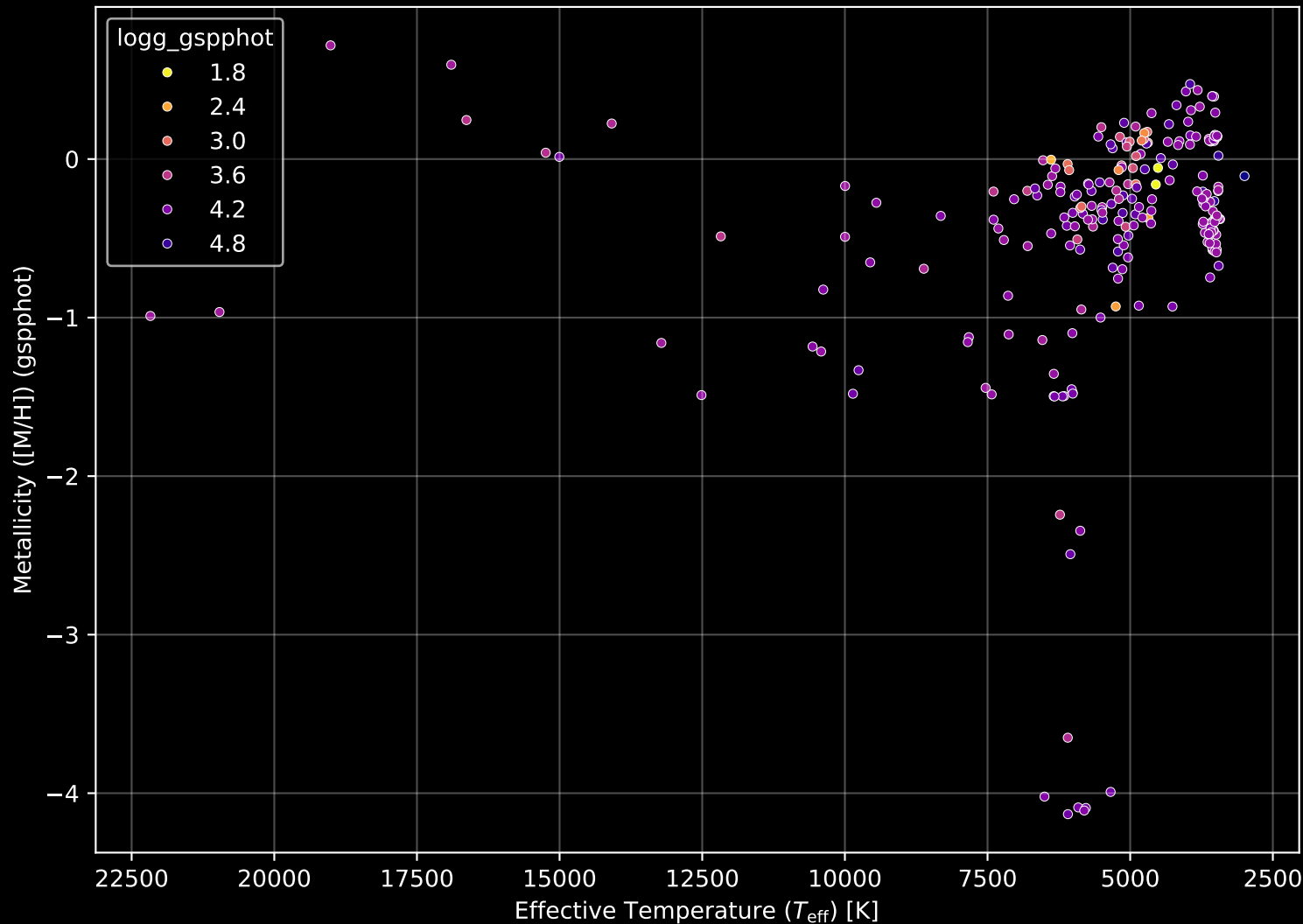
APOGEE DR17 Field: [ORIONC] Stellar Population Parameters (n= 236)
